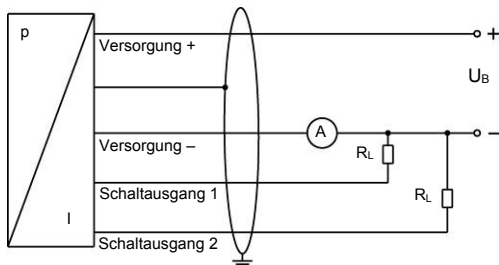
2-Leiter-System (Strom)
