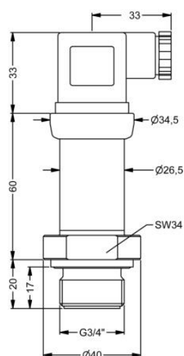
G 3/4" frontbündig DIN 3852
