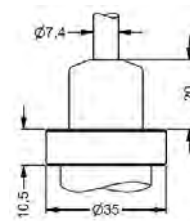
Kabelausgang, Kabel mit Belüftungsschlauch (IP 68) 9
