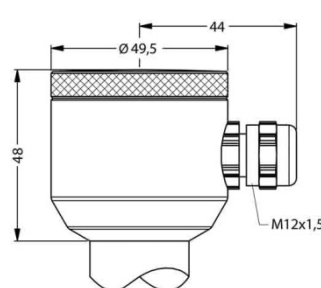
Kompakt-Feldgehäuse (IP 67)
