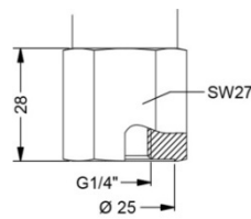
G 1/4" DIN 3852 Innengewinde
