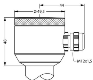
Kompakt-Feldgehäuse (IP 67)
