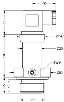
G1" frontbündig DIN 3852
