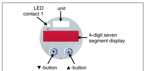
Fig. 4 Touchpad
