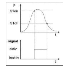
Fig. 5 hysteresis mode
