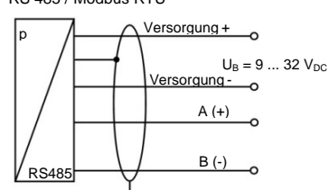
Abb. 2 Anschlusschaltbild
