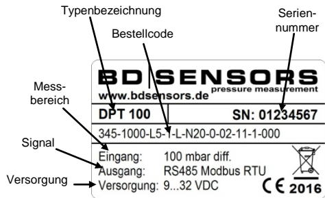
Abb. 1 Typenschild
