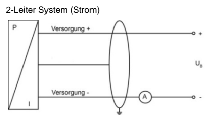
Abb. 2 Anschlussschaltbild
