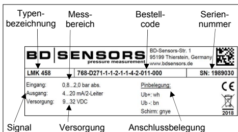
Abb. 1 Typenschild
